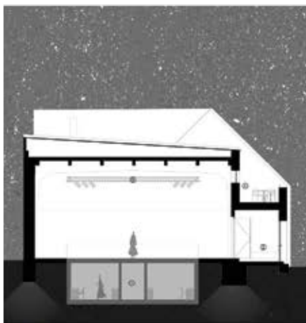
Rez B-B 1:100
